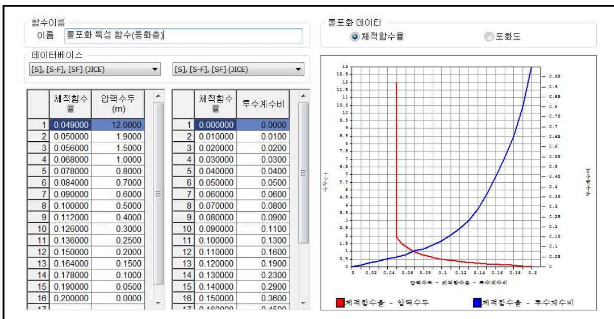
【그림 30.15】 압력수두-채적함수(포화도)-투수계수비 함수
